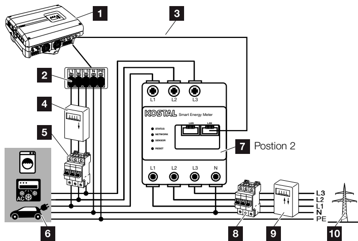
Abb. 66: Anschluss Energiezähler
