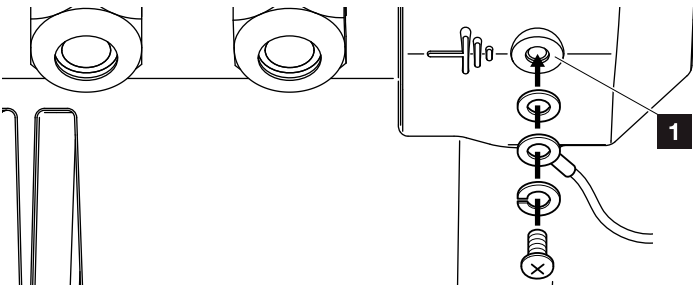
Abb. 24: Länderspezifischer PE-Anschluss
