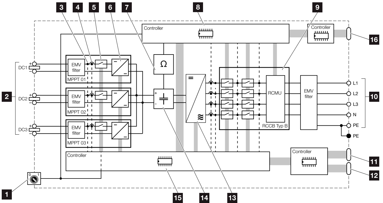
Abb. 65: Blockschaltbild
